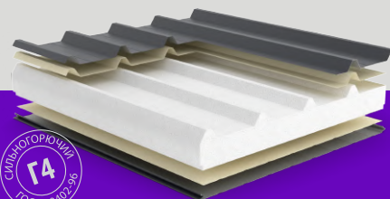
Пенополистирол (ПП)
