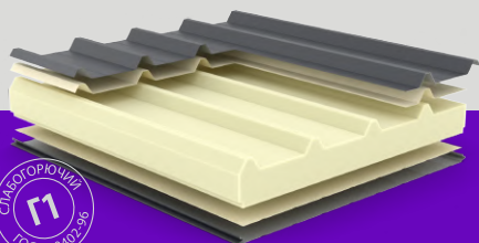
Пенополиизоцианурат (ПИР)
